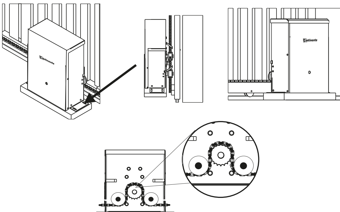
Figura 03: Transpassar a corrente conforme imagem e fixar no portão, com um ponto de solda, observando que a engrenagem se encaixe na corrente, para que ocorra a movimentação do portão no momento que o movimentador for acionado.
